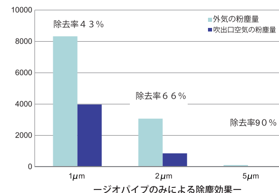
ージオパイプのみによる除塵効果ー
