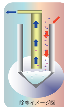
除塵イメージ図
